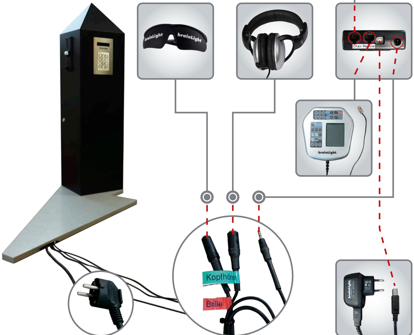
Steuerungsbox: Siehe rechts unten an der Basis der Sesslerückseite
